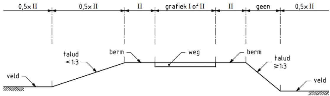
Figuur C.16 — Overzicht in rekening te brengen aslaststelsels
